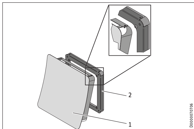
1 Schallschutz-Innenblende
